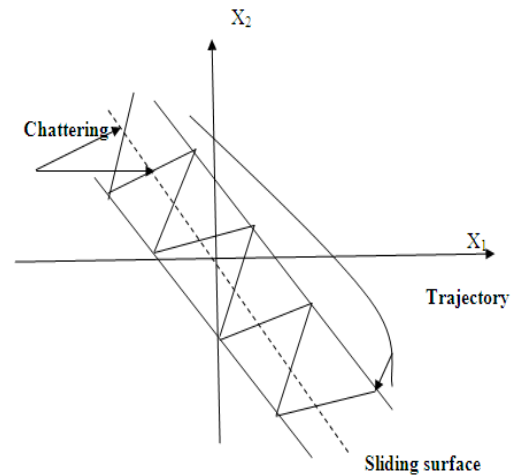
Fig. 4: Chattering
