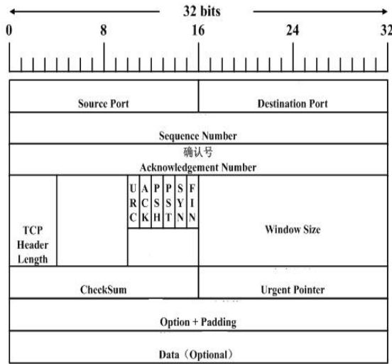
Fig. 3: The TCP format
