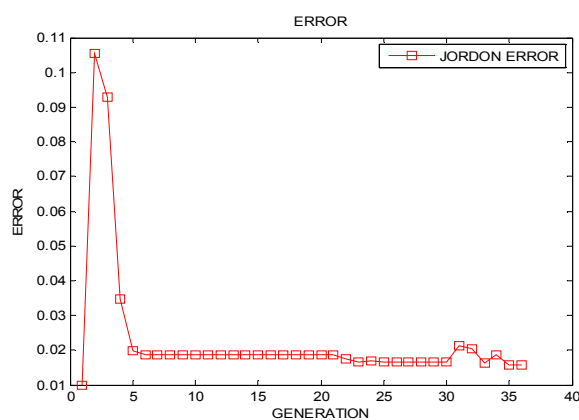
Fig. 8: GA-JNN error
