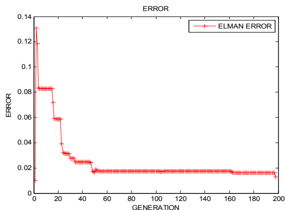
Fig. 6: GA-BPNN error
